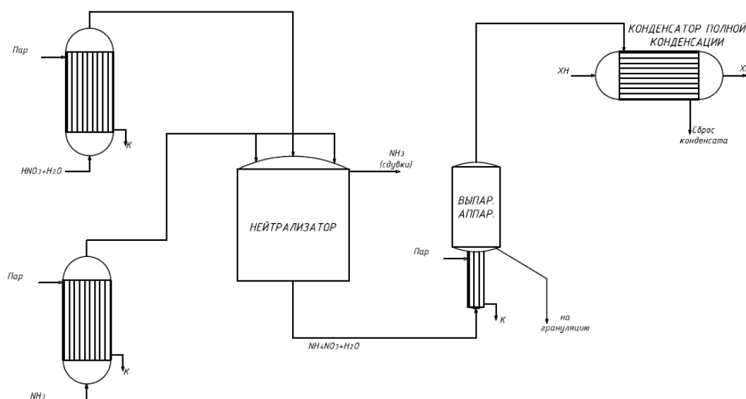
Рисунок 3 – Технологическая схема
