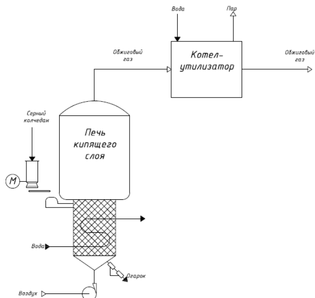
Рисунок 1 – Технологическая схема
